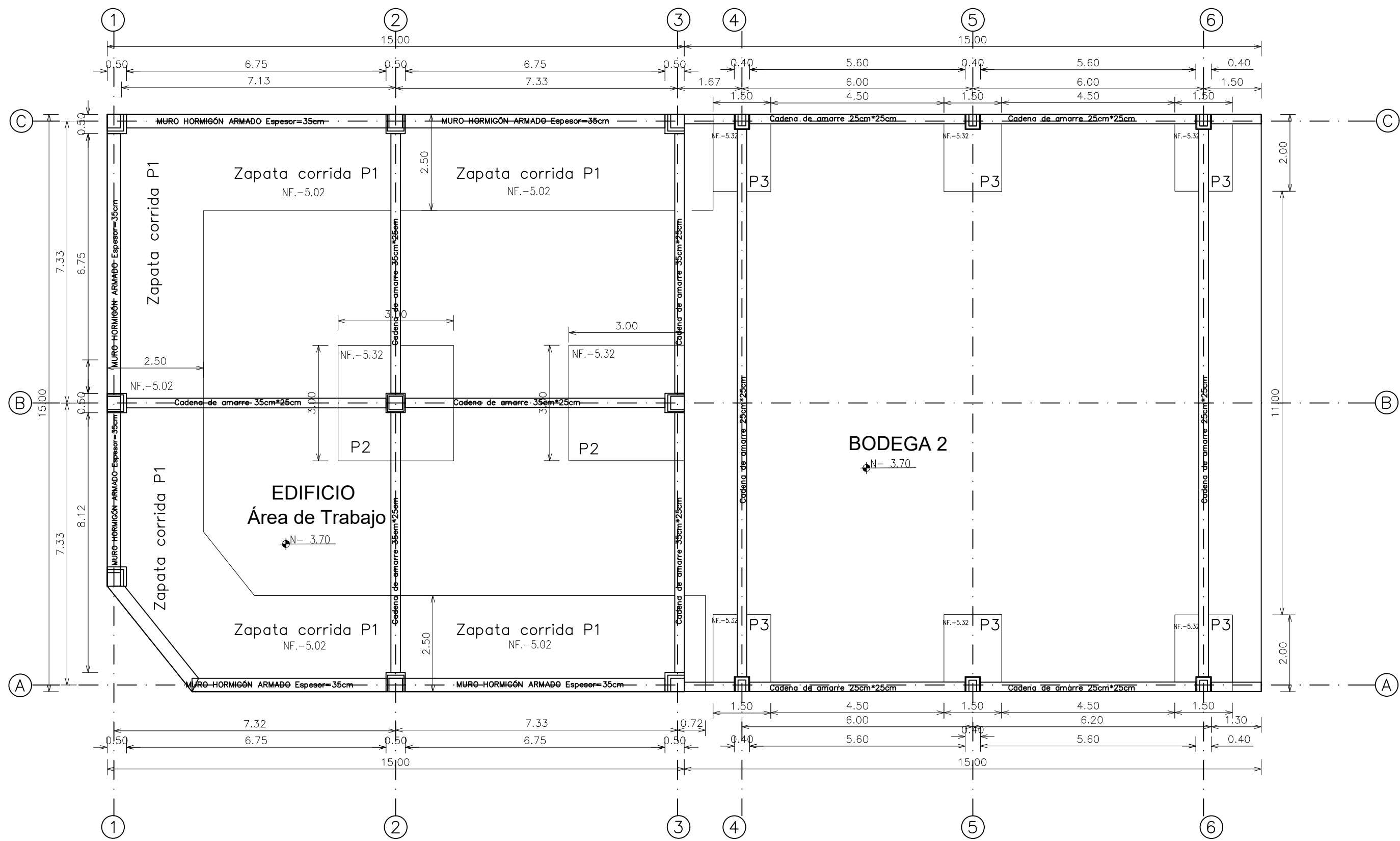
PLANTA CIMENTACIÓN Escala 1:100
