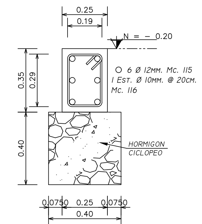
DETALLE DE CADENA CORTE 1-1 Escala 1:12.5
