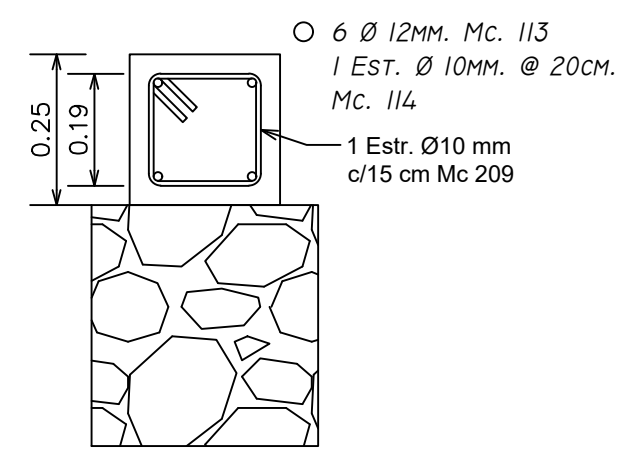
DETALLE DE CADENA CORTE 2-2 Escala 1:12.5
