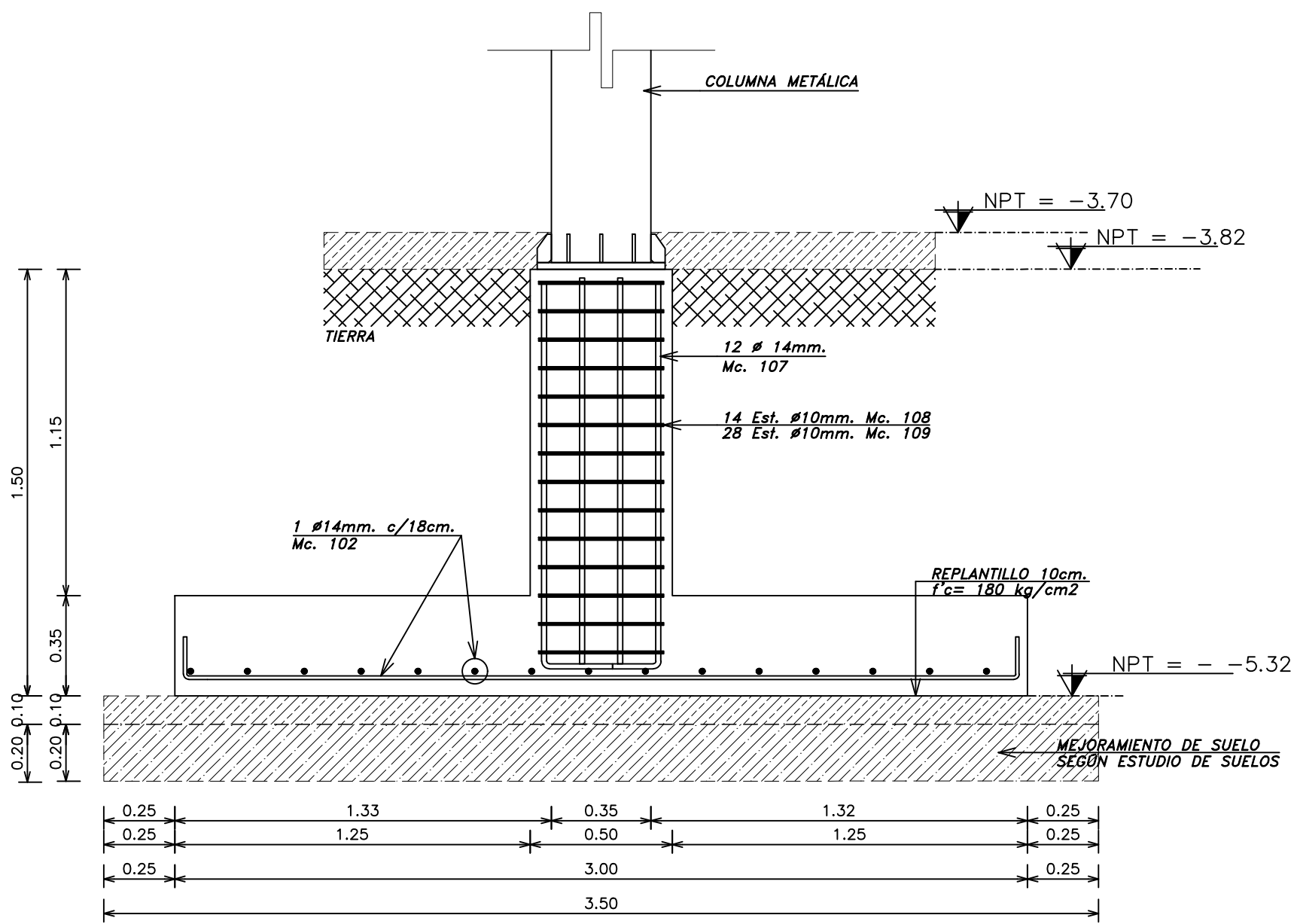
DETALLE DE ELEVACIÓN DE CIMENTACIÓN P2 (2 unidades) Escala 1:20
