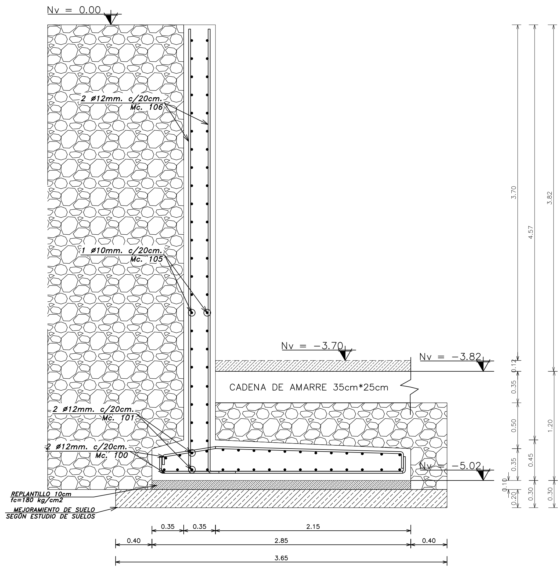
DETALLE DE MURO-ZAPATA CORRIDA P1 Escala 1:25
