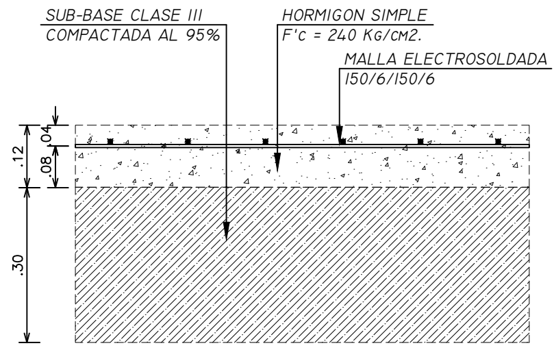
DETALLE DE CONTRAPISO NORMAL Escala 1:10
