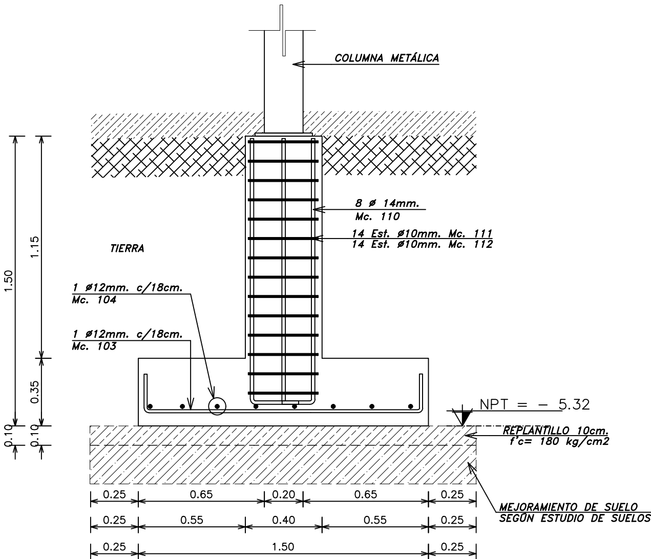
DETALLE DE ELEVACIÓN DE CIMENTACIÓN P3 (6 unidades) Escala 1:20
