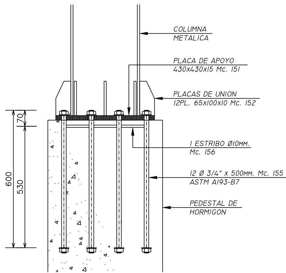
ELEVACION TIPICA DE CANASTILLAS Escala 1:10
